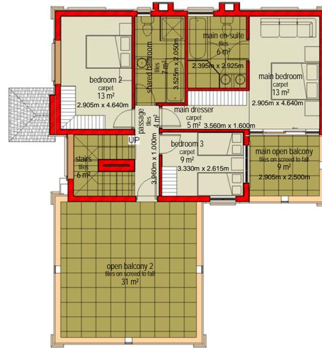
2 03 first 1 : 100
